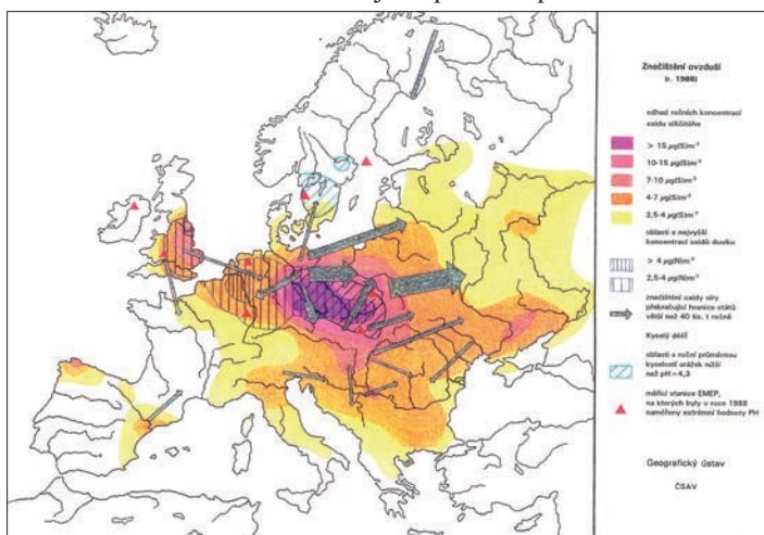
Mapa emisí oxidu siřičitého v Evropě koncem 80. let minulého století
